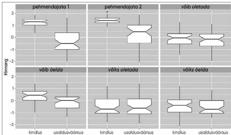
Joonis 3. Autori kindlusele ja väite usaldusvärsusele antud hinnangute võrdlus (z-skoorid).
