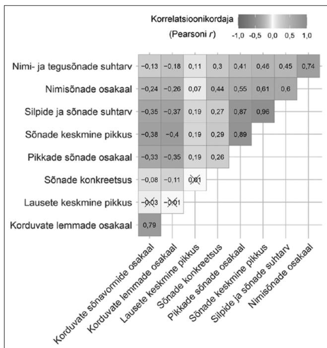
Joonis 2. Komplekskuse mõõdikute vahelised korrelatsioonid. Statistiliselt ebaolulised korrelatsioonid on märgitud X-iga.
