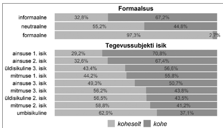
Joonis 1. Vormide koheselt ja kohe jaotumine vastavalt kahe statistiliselt olulise tunnuse tasemele.
